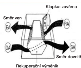
Režim s rekuperací tepla
