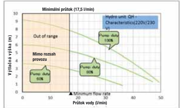
Charakteristika čerpadla HWS-(P)1404XWH (11,14,16 kW)
